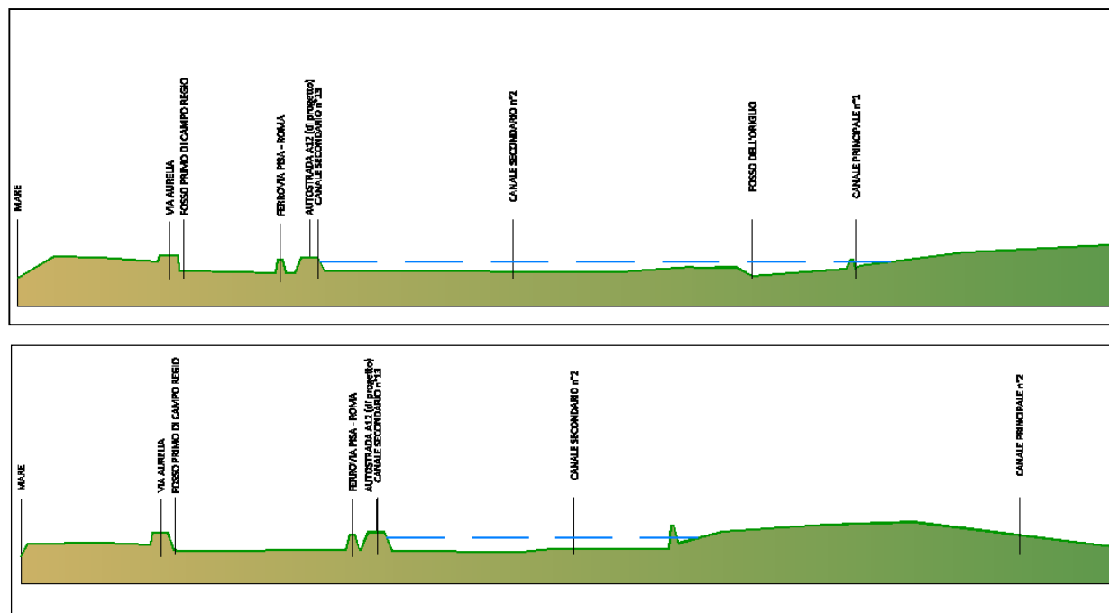
Sezioni territoriali Est-Ovest della soluzione luglio 2013, con indicato il massimo livello di allagamento, corrispondente all'evento critico del novembre 2012.
