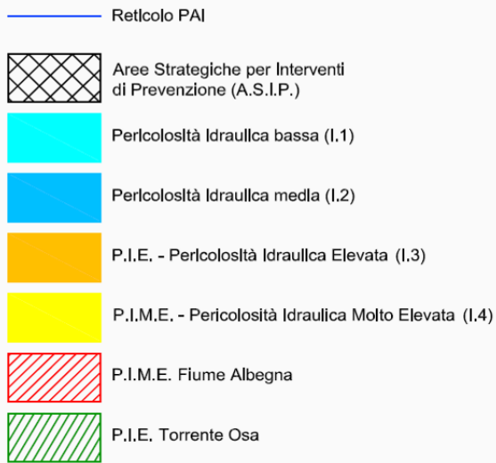
Figura 9 Stralcio della Carta delle pericolosità idrauliche del comune di Orbetello – Fonte: Tav. 50A del Regolamento Urbanistico di Orbetello
